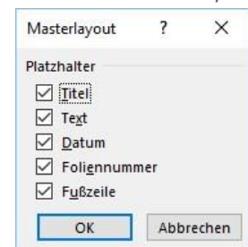
Abbildung 3 - Dialogfenster Masterlayout
