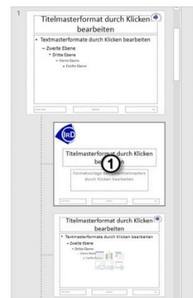
Abbildung 3 - Dialogfenster Masterlayout
