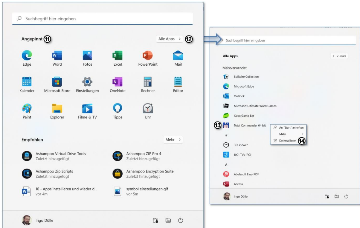
Abbildung 4 - Apps deinstallieren
