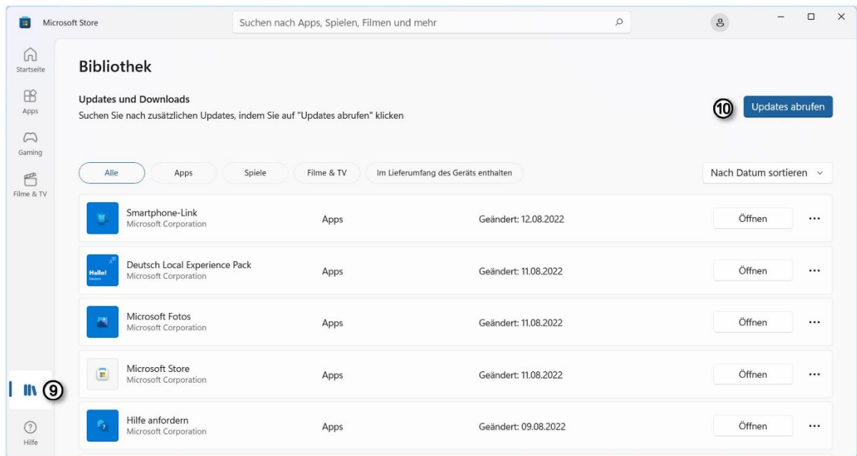
Abbildung 3 - Apps aktualisieren
